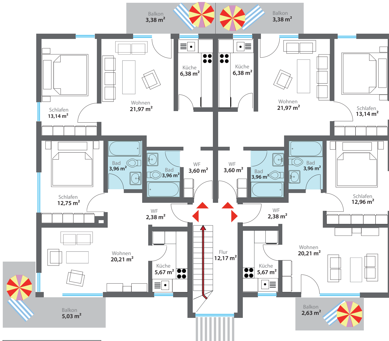
Grundriss OG
